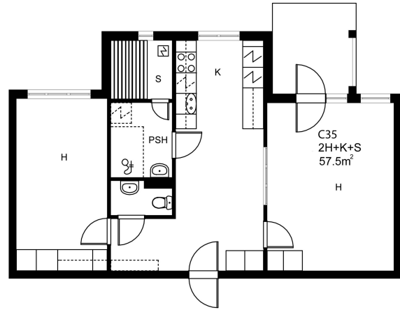
Pohjakuva suuntaa antava, ei mittakaavassa © virtualdesign.fi
